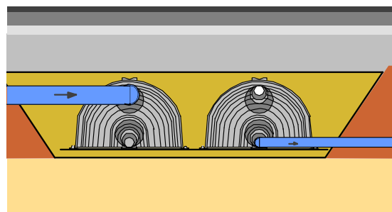
Fig. 3: Rainwater attenuation
